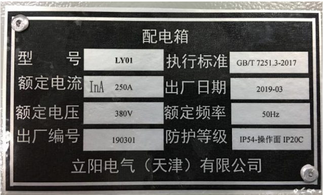
铭牌照片
