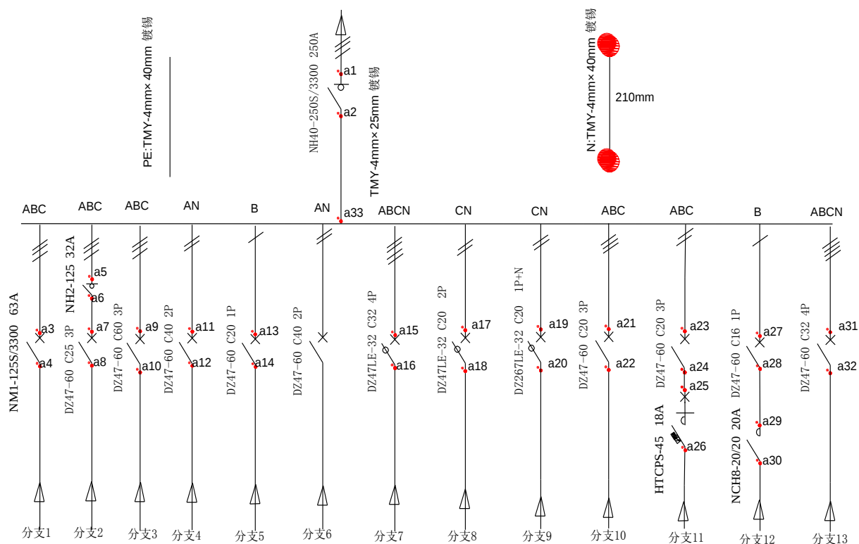
温升示意图、温升参数表、母排绝缘支撑件及绝缘夹板的安装布置图 F1:
