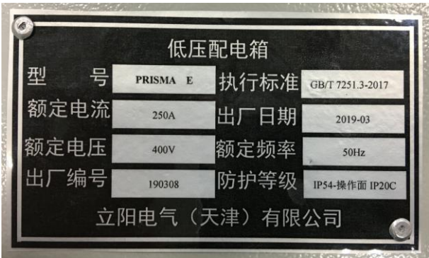
铭牌照片
