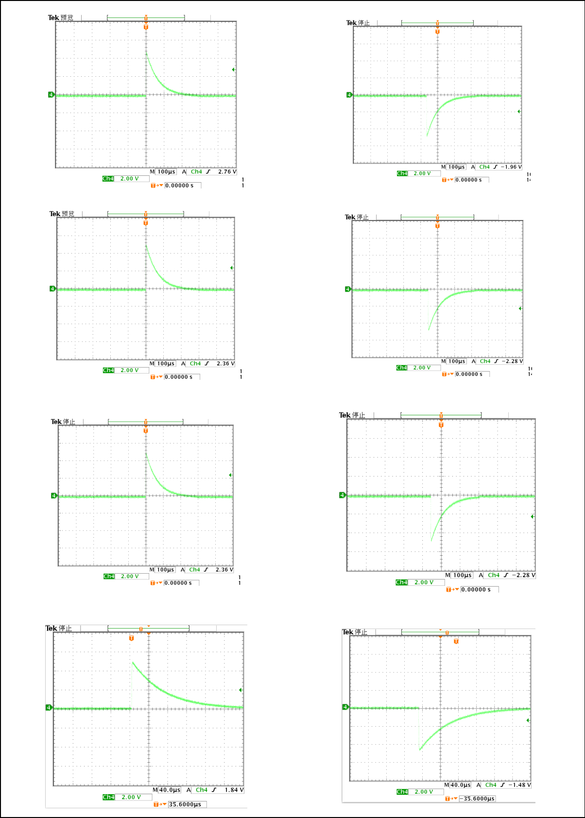
冲击耐受电压示波图
