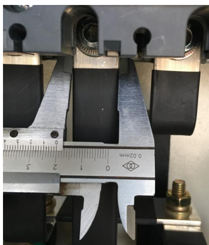
主开关进出线宽度照片
