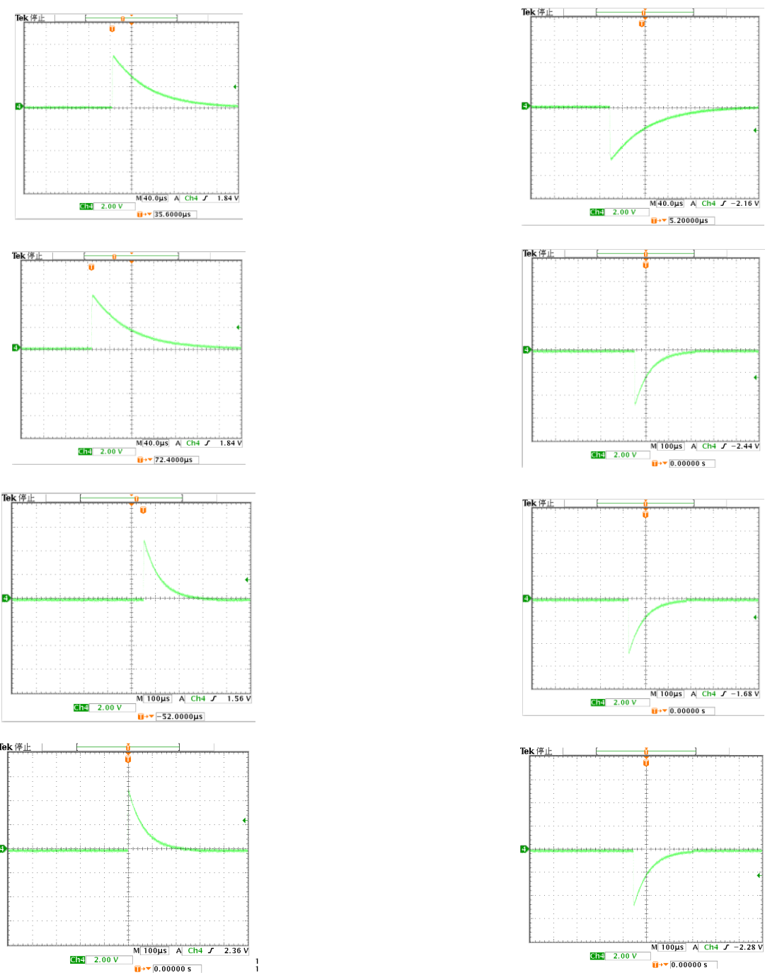
冲击耐受电压示波图
