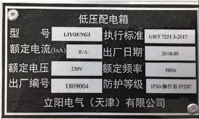
铭牌照片
