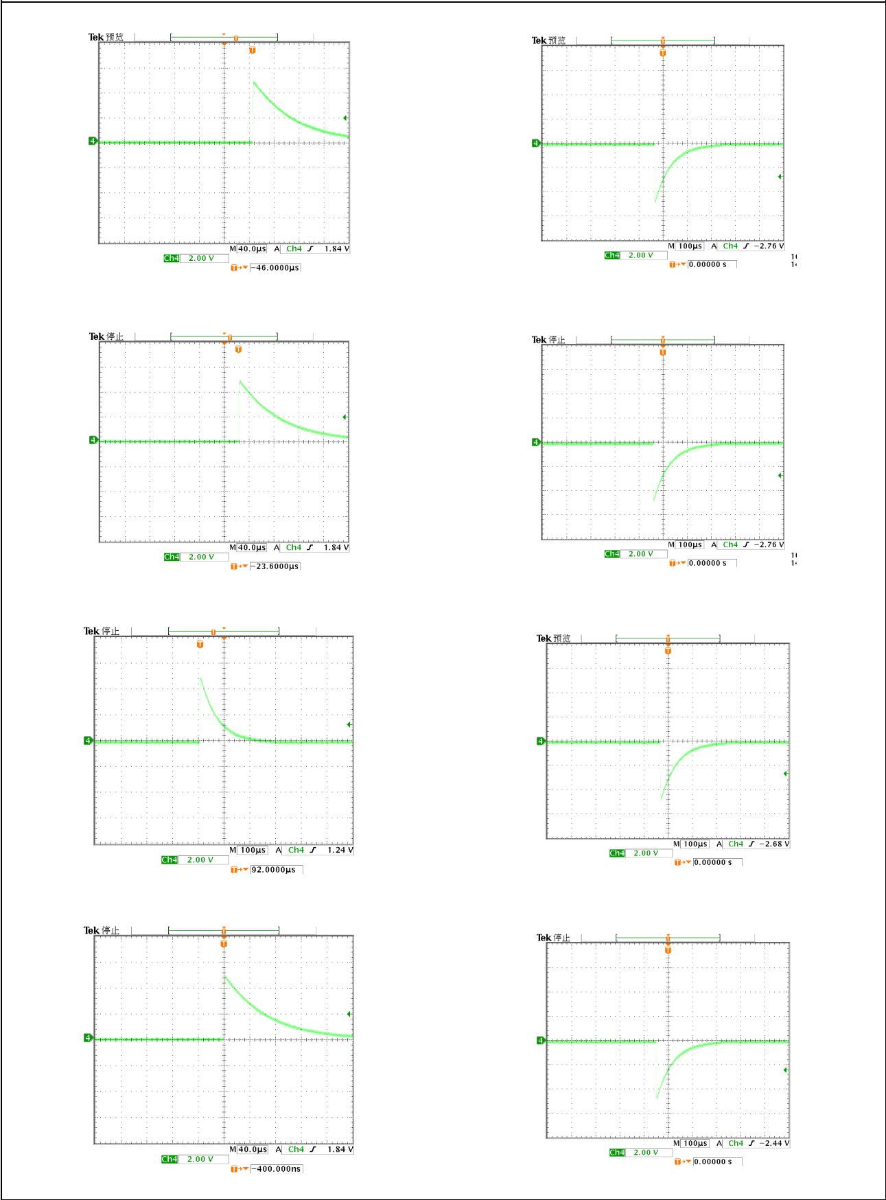
冲击耐受电压示波图
